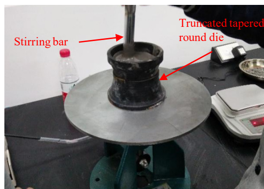
图3 水泥胶砂流动度仪
