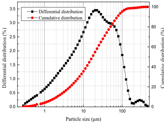
图 1 尾矿粒度分析结果
