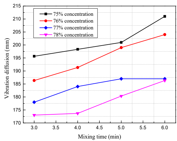
图 7 不同质量分数条件下膏体振动扩散度与搅拌时间关系图
