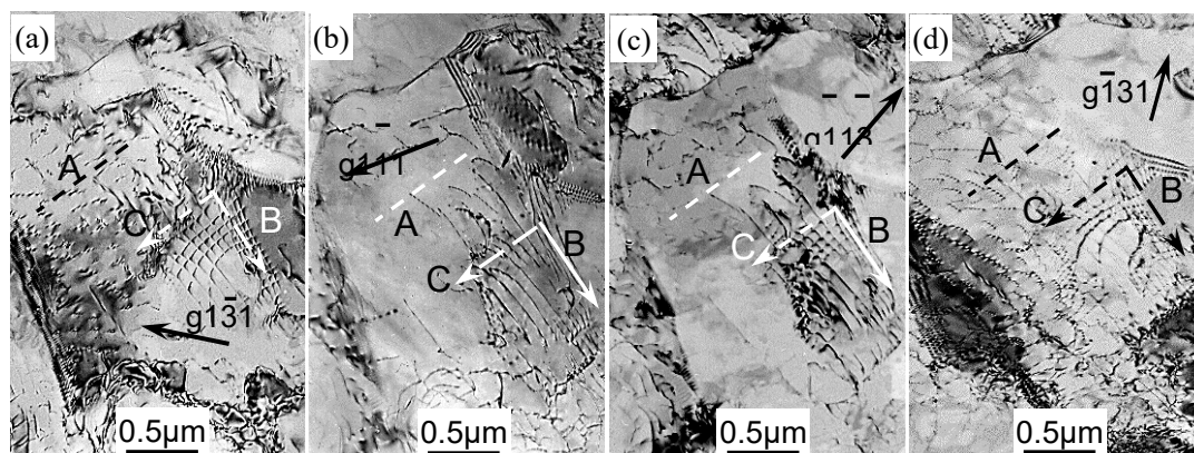
图 8 合金经 800℃/220MPa 蠕变断裂后的位错组态
