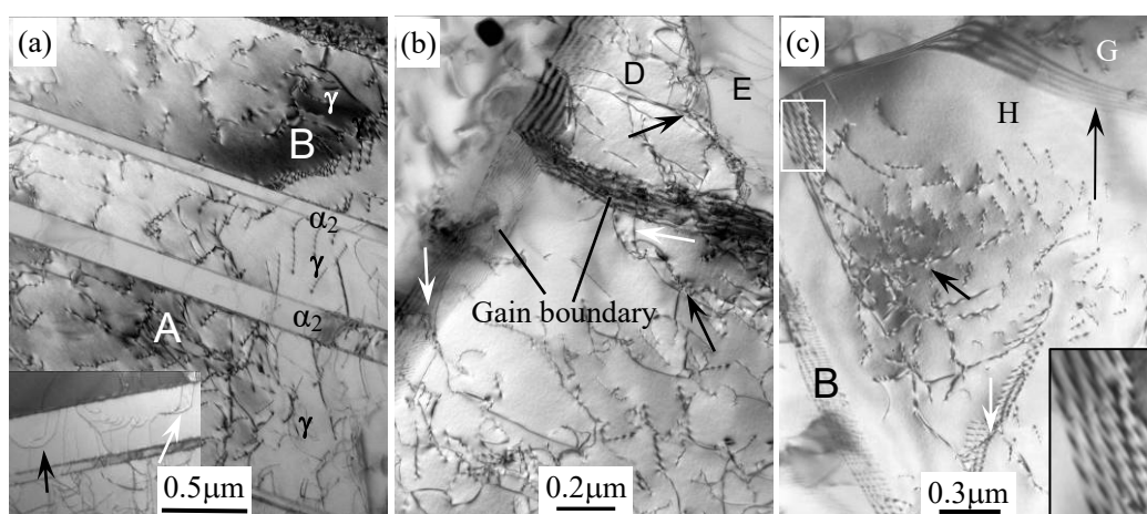
图 7 锻造态合金经 800℃/220MPa 蠕变断裂后的组织形貌
