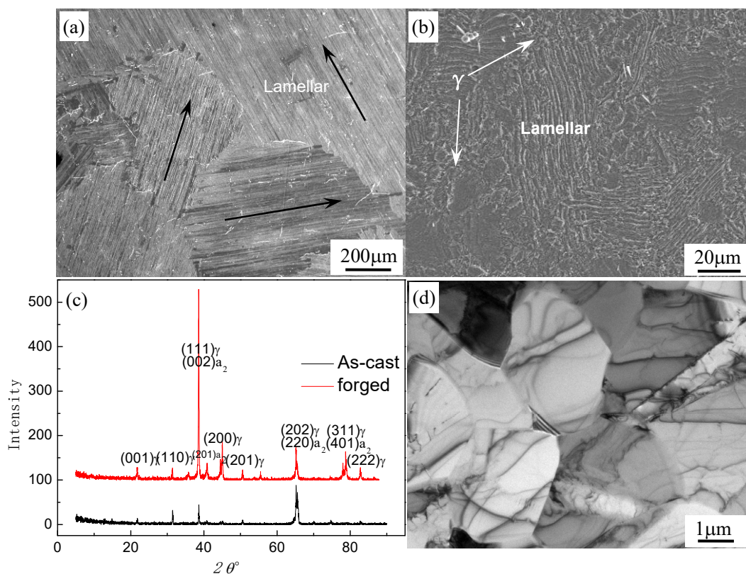
图 1 铸造态与锻造态高 Nb-TiAl 合金的组织形貌及 XRD 图谱
