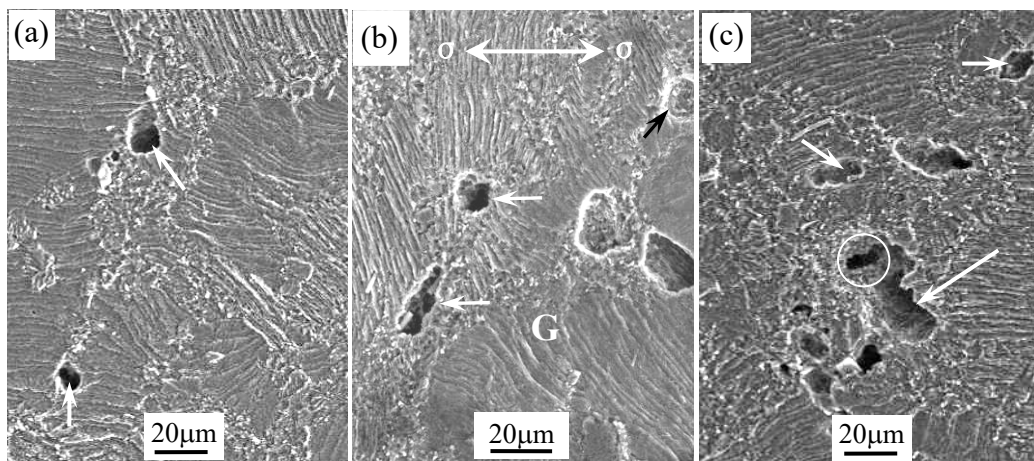
图 9 锻造态合金经 800^\circ\text{C}/220\ \text{MPa} 蠕变断裂后，裂纹沿晶界的萌生与扩展
