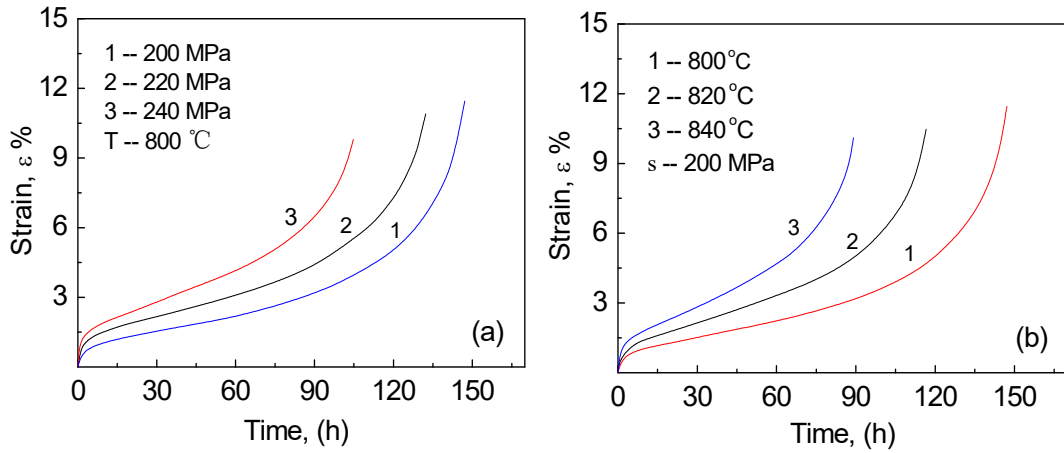
图 3 锻造态合金在不同条件测定的蠕变曲线
