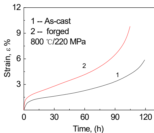
图 2 铸造态与锻造态高 Nb-TiAl 合金在 800°C/220MPa 条件下的蠕变曲线
