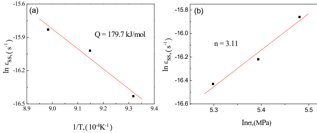
图 4 锻造态合金在近 800℃中期蠕变期间应变速率与施加温度、应力的关系
