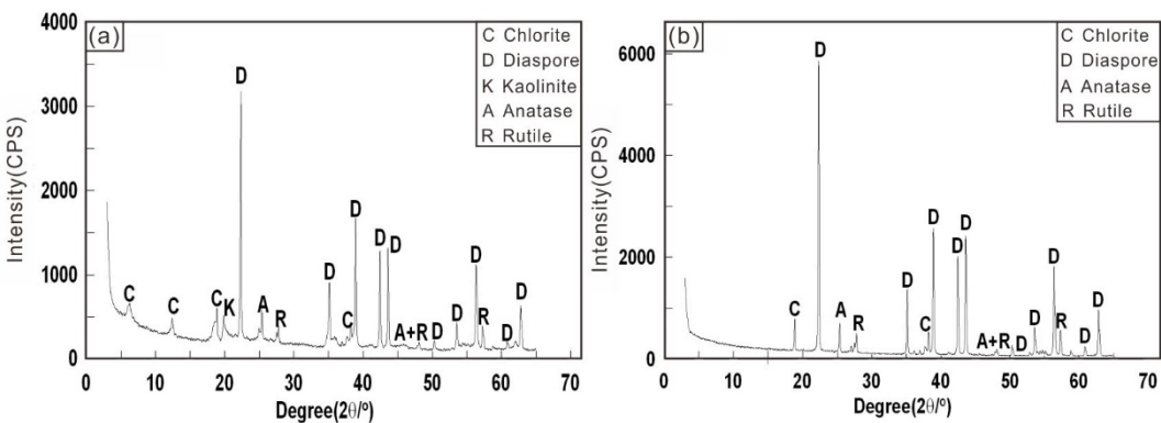
图 5 铝土矿 XRD 矿物图谱
