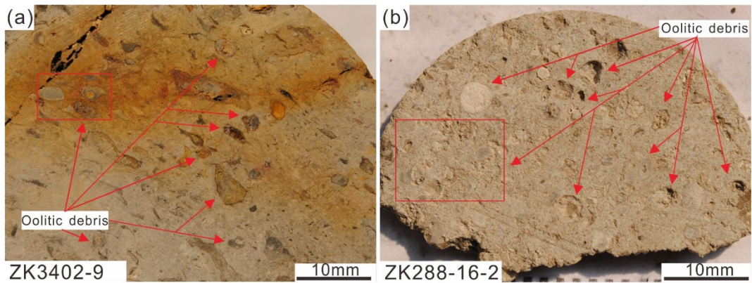
图 9 鲕粒残骸
