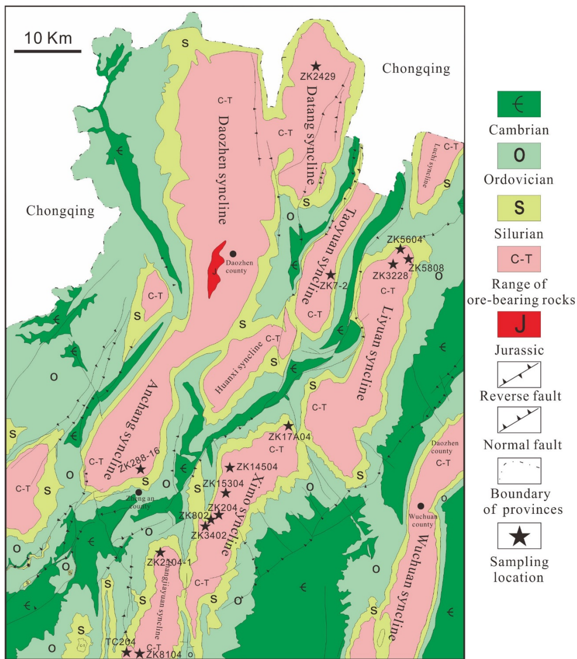
图 1 研究区地质图（据文献[13], [21]修改）
