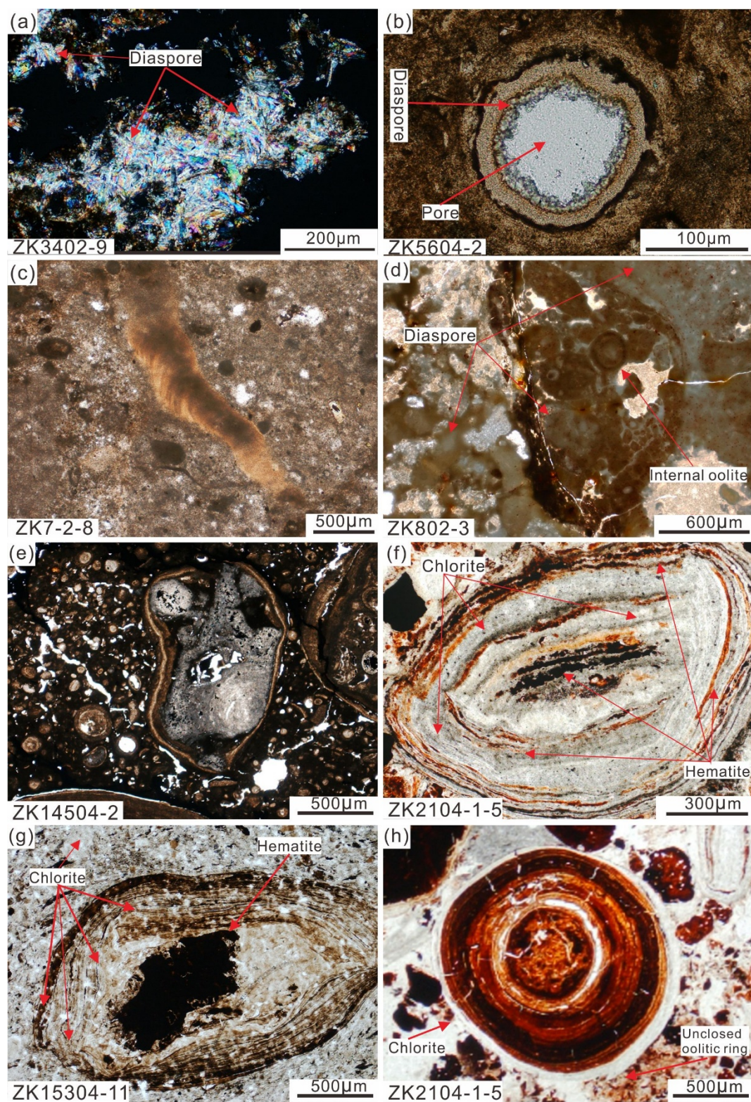
图 6 铝土矿镜下特征
