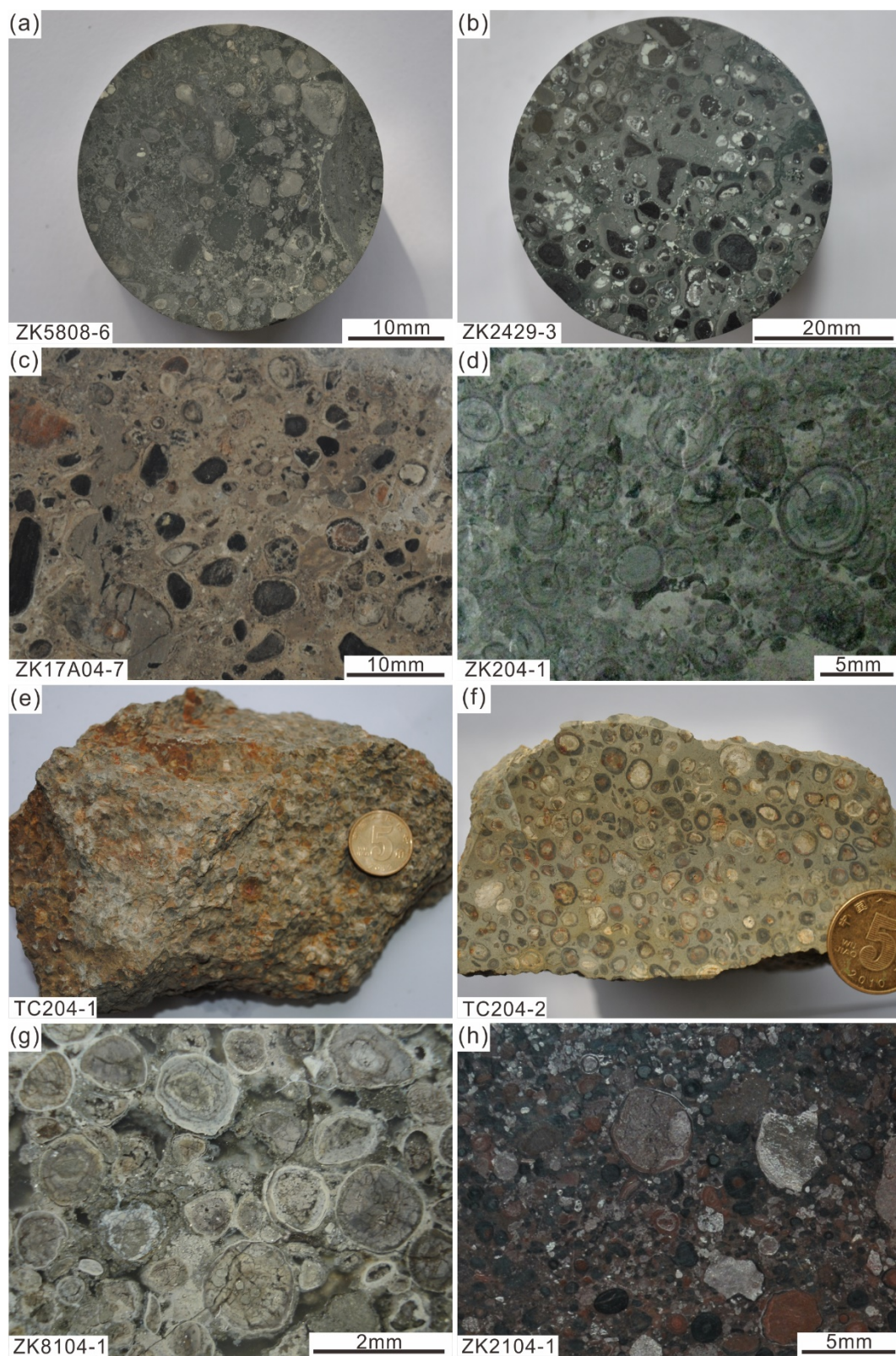
图2 手标本与岩心中的鲕粒((c)引自文献 [14]; (h)引自文献[27])
