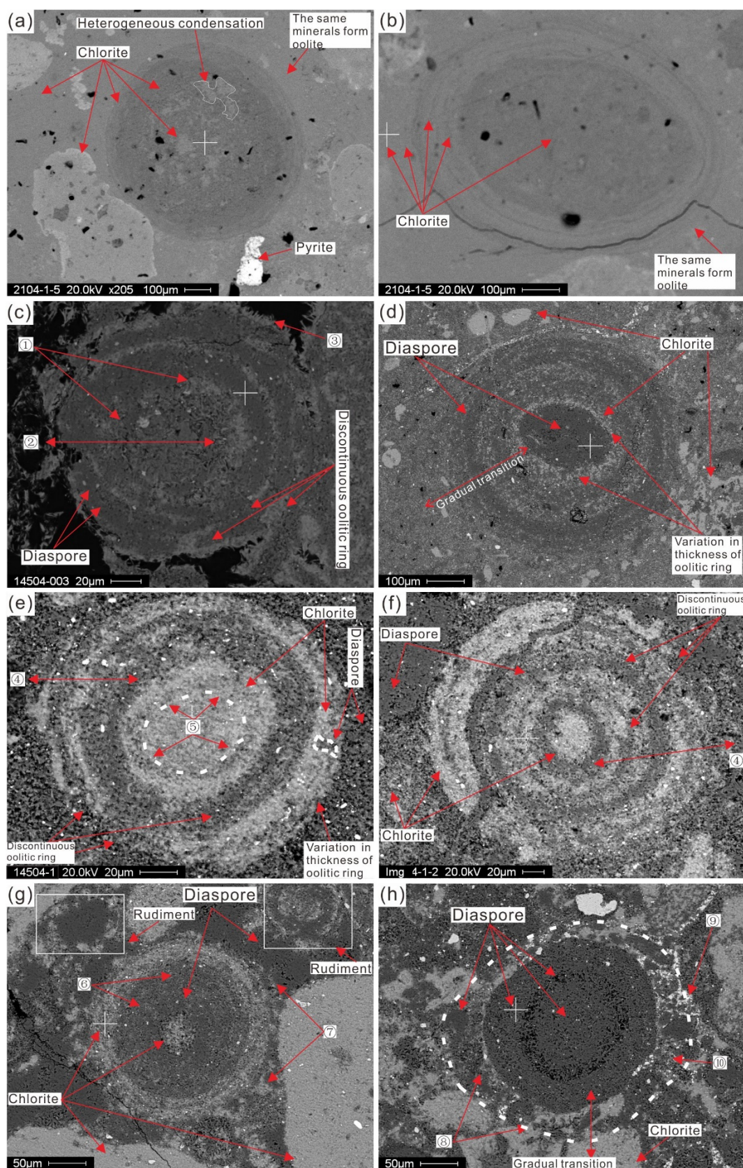
图 4 鲕粒形态特征 (扫描电镜照片)
