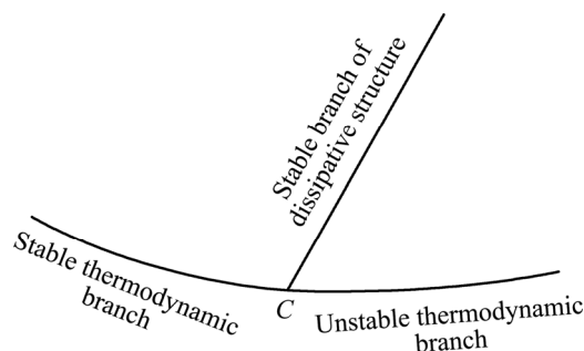
图 3 过临界点 C, 热力学分支失稳, 系统要进入稳定的耗散结构分支或不稳定的热力学分支
