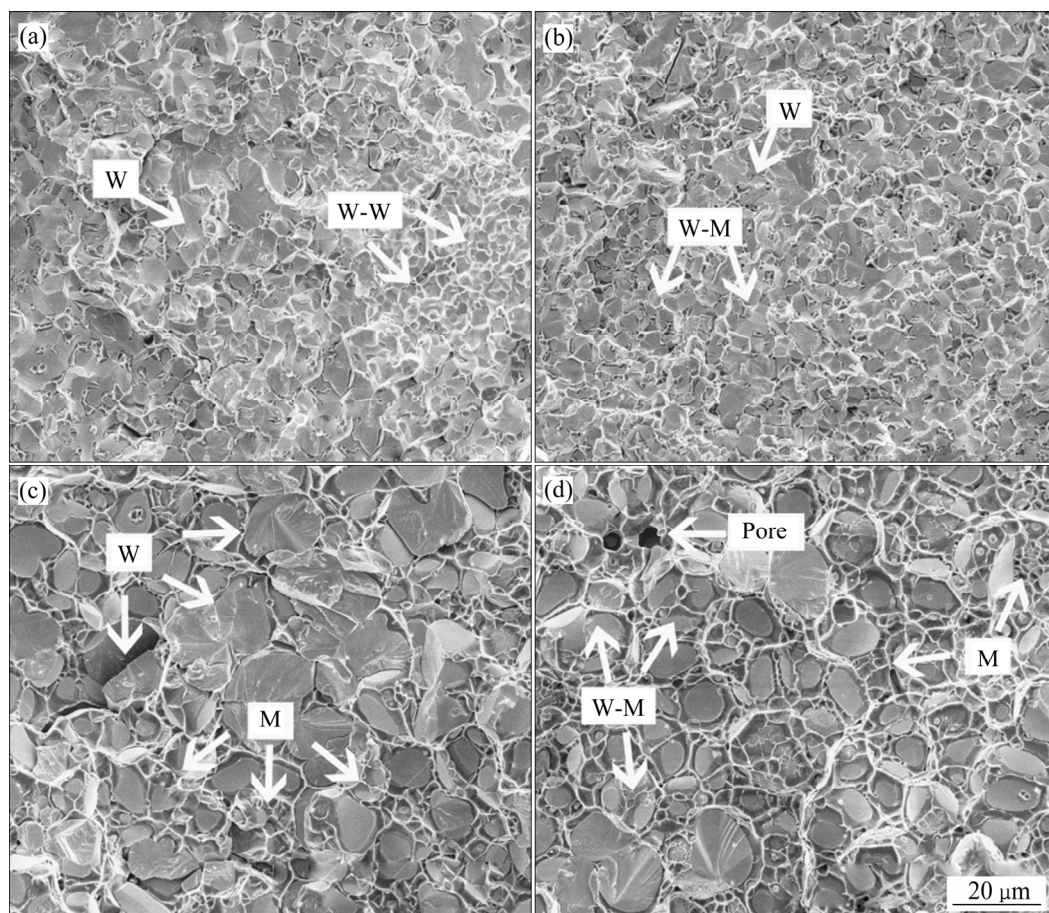
图 7 不同铜含量钨合金断口形貌图
