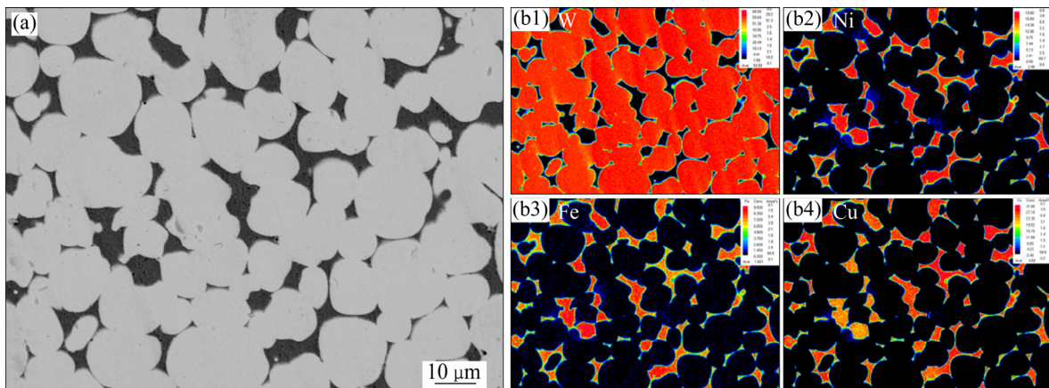
图 4 90W-4.2Ni-1.8Fe-4Cu 合金微观组织形貌
