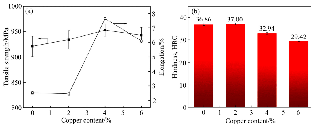
图 5 不同铜含量热等静压钨合金的抗拉强度、伸长率和硬度
