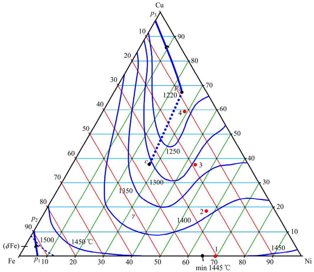
图 2 Ni-Fe-Cu 三元液相线投影图 [13] Fig 2 Liquidus surface projection of Ni-Fe-Cu [13] : 1—90W-7Ni-3Fe; 2—90W-5.6Ni-2.4Fe-2Cu; 3—90W-4.2Ni-1.8Fe-4Cu; 4—90W-2.8Ni-1.2Fe-6Cu
