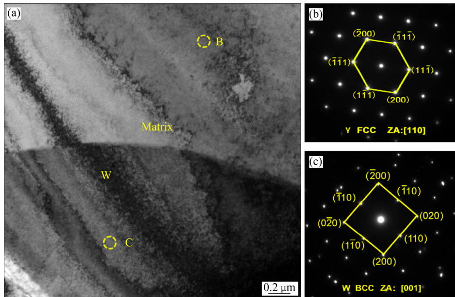
图 3 90W-4.2Ni-1.8Fe-4Cu 合金 TEM 图像以及选区电子衍射
