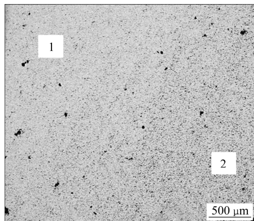
图 6 热等静压 90W-2.8Ni-1.2Fe-6Cu 合金的微观组织
