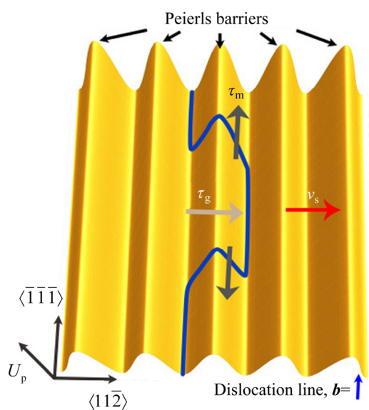
图1 低温下 BCC 钨中螺型位错扭结对在(110)平面上传播的示意图 [13]
