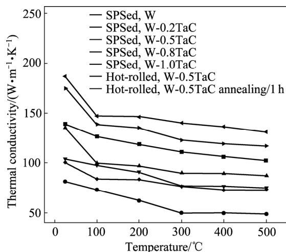
图 5 不同状态 W-TaC 合金热导率与温度的变化关系 [46]
