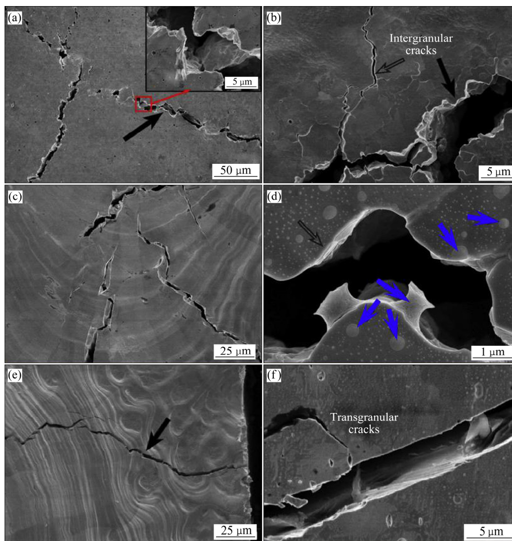
图 7 不同功率密度热负荷加载后轧制态和锻造态 W-ZrC 样品表面 SEM 像 [52]
