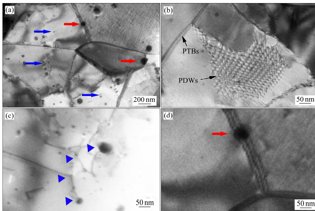
图 3 透射图像下轧制态 W-HfC 合金中 HfC 颗粒和位错的分布状态 [30]
