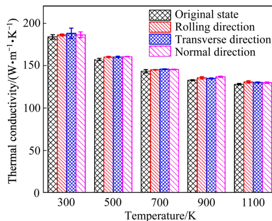
图 6 热轧 W-Y 2 O 3 合金沿不同轧制取向热导率与温度的变化关系 [48]
