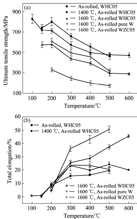
图 2 不同状态纯 W, W-HfC 合金和 W-ZrC 合金的高温拉伸屈服强度和伸长率 [30]
