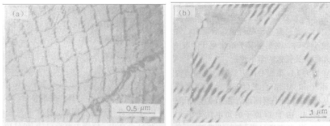
图2 TiAl+Ga三元合金的典型变形亚结构
