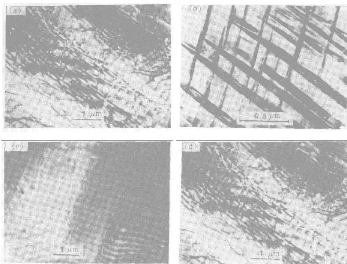
图3 具有较好室温延性的TiAl基合金的典型变形亚结构
