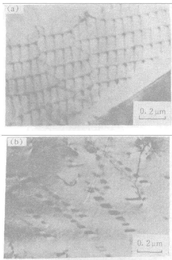
图1 Ti-36Al(Ti50Al50)合金的典型变形亚结构
