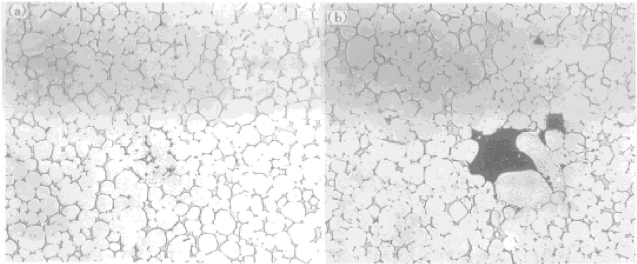
图3 经1530℃液相烧结2h, PIM与传统PM的合金的孔隙比较(×100, 未腐蚀)
