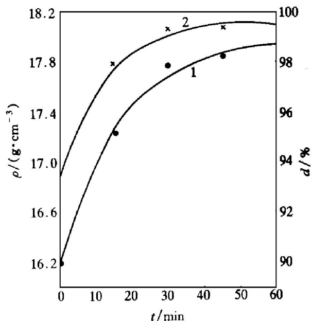
图 1 在 1530 ℃液相烧结时, 烧结密度与保温时间的关系
