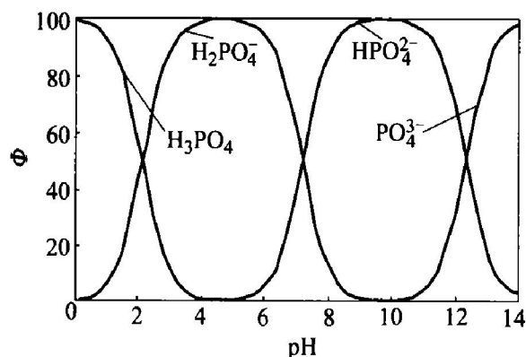
图 5 (\text{NaPO}_3)_6 溶液中各水解组分的 \Phi (分布系数)-pH 值关系图
