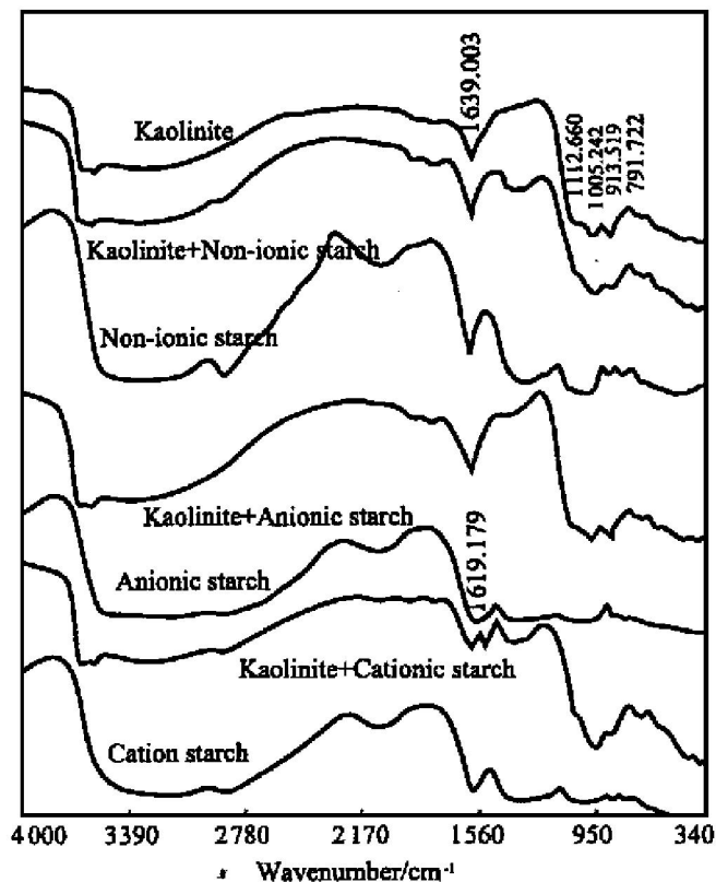
图 5 药剂和高岭石作用前后的红外光谱
