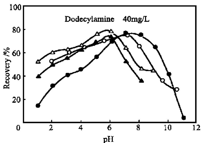
图 1 矿浆 pH 值对一水硬铝石可浮性的影响
