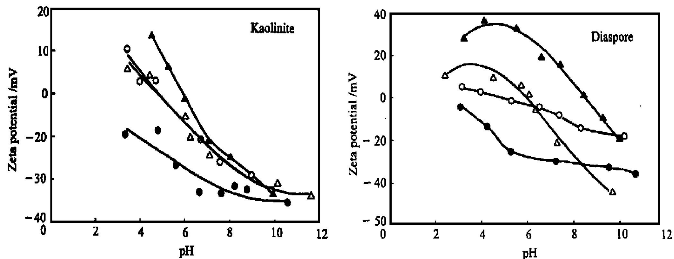
图 3 矿物的 \zeta -电位与 pH 值的关系
