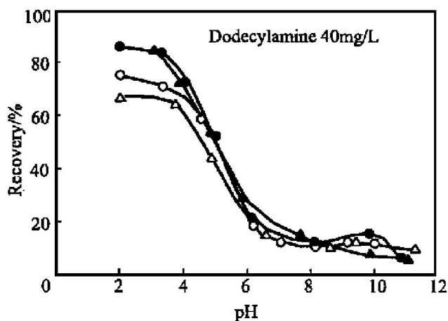
图 2 矿浆 pH 值对高岭石可浮性的影响
