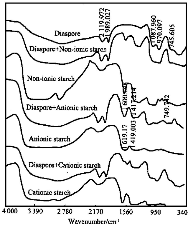
图 4 药剂和一水硬铝石作用前后的红外光谱图
