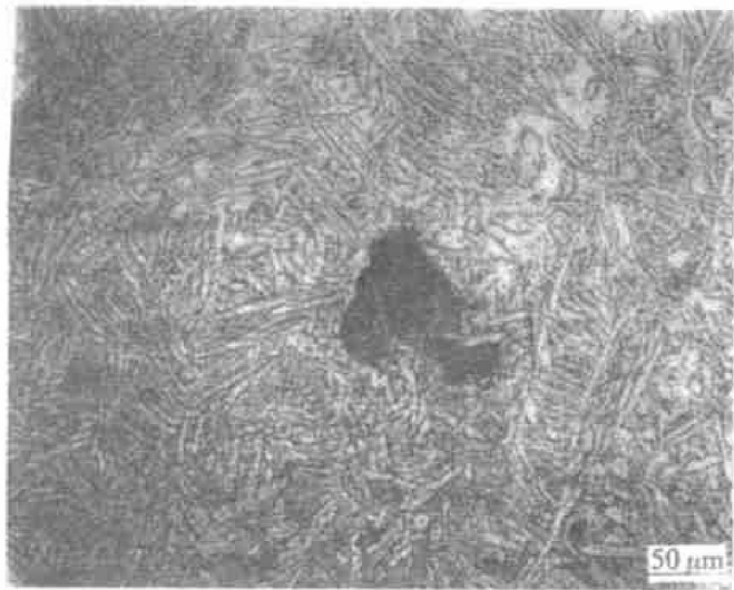
图 3 试样 5AS1N 点蚀后的形貌
