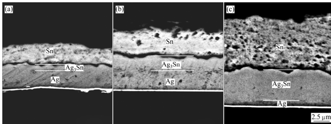
图 5 经不同温度和时间热处理后 Ag/Sn 偶的截面背散射电子像
