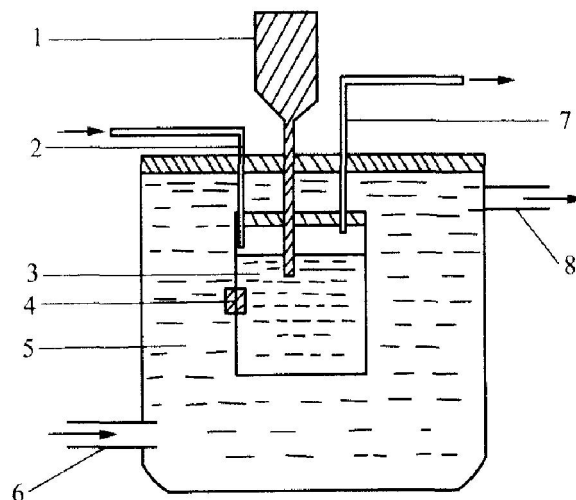
图 1 超声处理装置示意图
