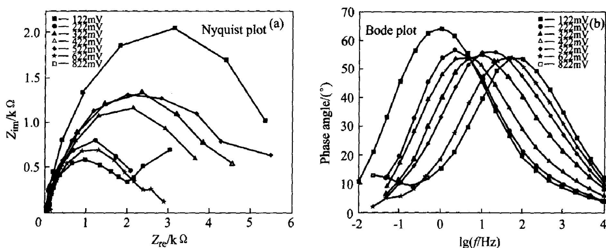
图 5 脆硫锑铅矿电极在含 0.001 mol/L 乙硫氮的饱和 \text{Ca}(\text{OH})_2 溶液中的交流阻抗谱
