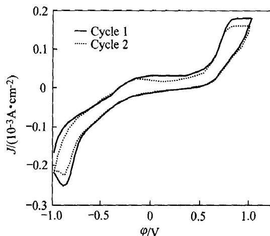
图 3 脆硫锑铅矿电极在含 0.001 mol/L 乙硫氮的饱和 Ca(OH) 2 溶液中的多次循环伏安图
