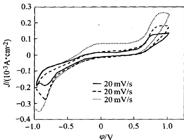
图 2 脆硫锑铅矿电极在 0.001 mol/L 乙硫氮 - 饱和 Ca(OH) 2 溶液中不同扫描速度时的循环伏安曲线
