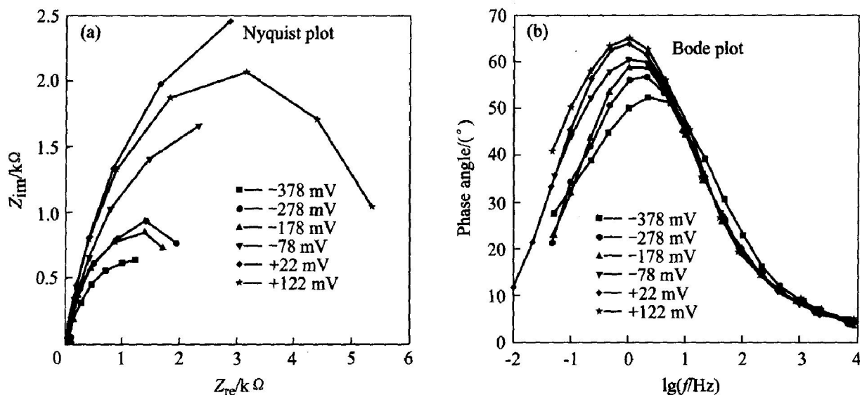
图 4 脆硫锑铅矿电极在含 0.001 mol/L 乙硫氮的饱和 \text{Ca}(\text{OH})_2 溶液中的交流阻抗谱
