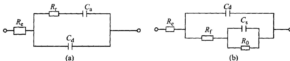
图 6 脆硫锑铅矿在含 0.001 mol/L 乙硫氮的饱和 \text{Ca}(\text{OH})_2 溶液中的等效电路
