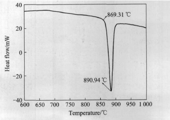
图 1 差热分析的 DSC 曲线 Fig. 1 DSC curve of CuMnCr alloy
