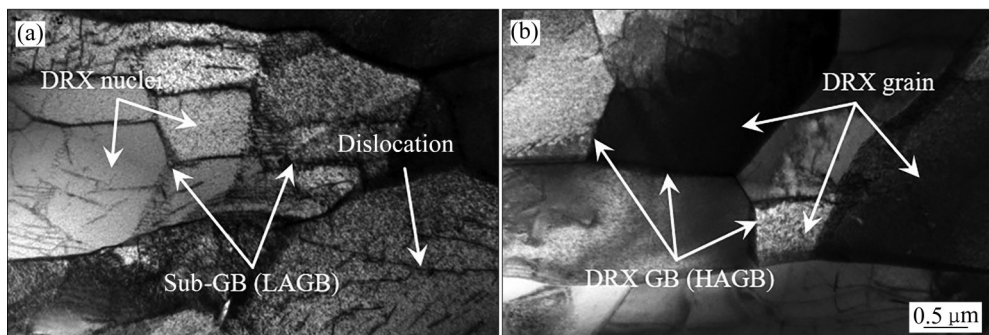
图 8 铸态 Ti-5553 合金在( 1100\text{ }^{\circ}\text{C} , 10\text{ s}^{-1} , 70%)变形后的 TEM 组织
