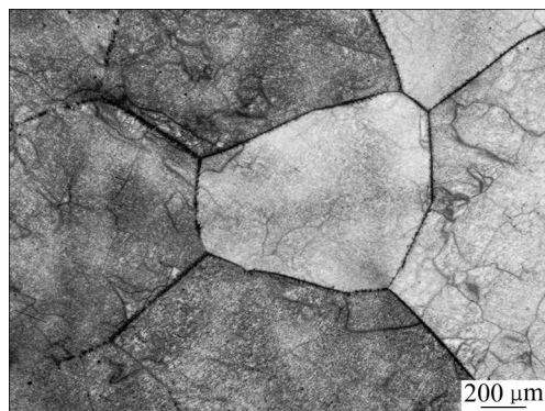
图1 铸态Ti-5553合金的金相组织
