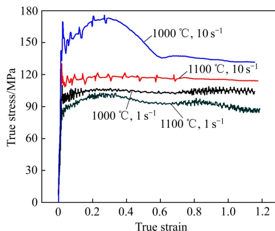
图3 铸态 Ti-5553 合金在不同变形温度和应变速率下的真应力-真应变曲线
