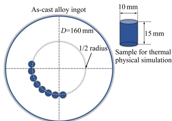
图2 铸态Ti-5553热模拟试样的取样位置示意图
