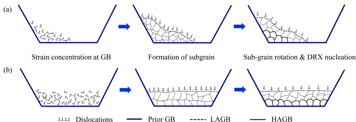
图9 铸态Ti-5553合金在高温高应变速率条件下的动态再结晶过程示意图
