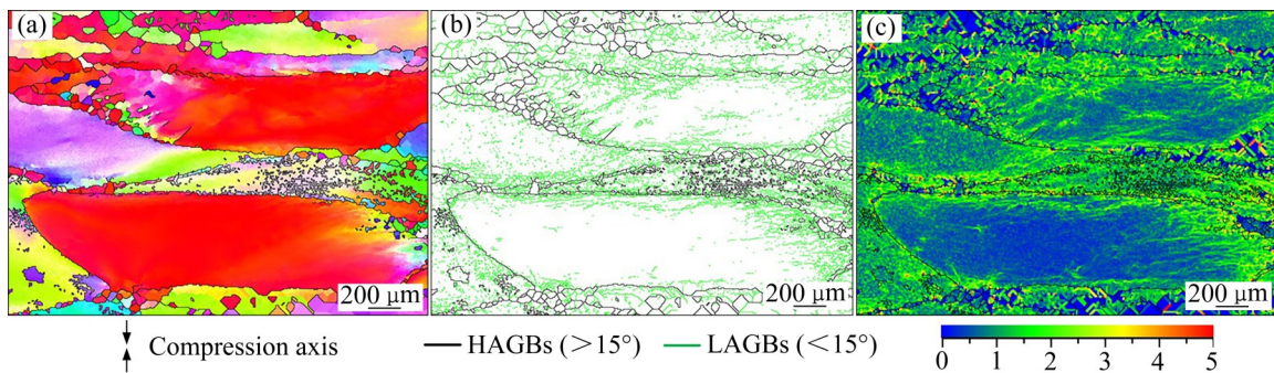
图 7 铸态 Ti-5553 合金在( 1100\text{ }^{\circ}\text{C} , 10\text{ s}^{-1} , 70%)变形后微观组织的 EBSD 表征结果
