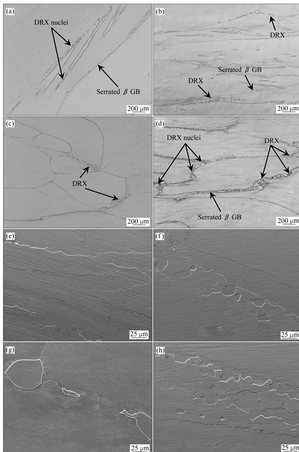
图5 铸态Ti-5553合金在 1100\text{ }^{\circ}\text{C} 条件下经不同应变速率和不同应变变量变形后微观组织(变形沿垂直方向进行)
