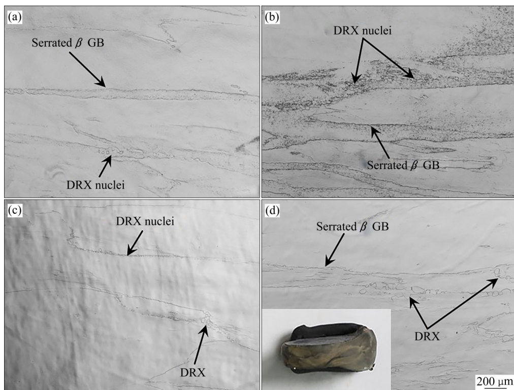
图4 铸态 Ti-5553 合金在1000 °C条件下经不同应变速率和不同应变量下变形后的微观组织(变形沿垂直方向进行)
