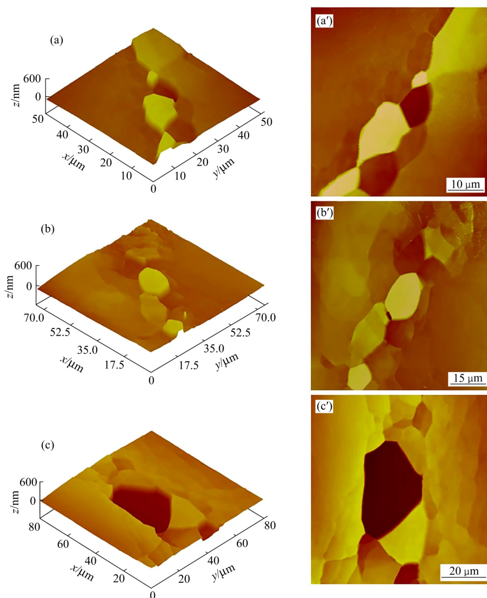
图6 铸态 Ti-5553 合金在不同条件变形后二维和三维 AFM 组织照片
