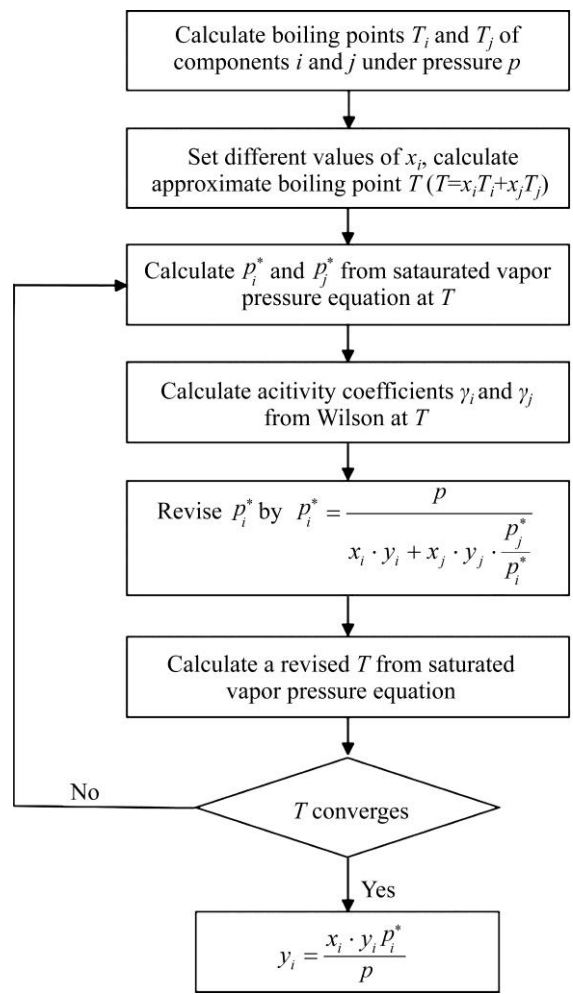
图 2 计算 Zn-Ni 二元合金体系 T - x - y 相图的流程图 Fig. 2 Flowchart of calculation T - x - y phase diagram of Zn-Ni binary alloy system
