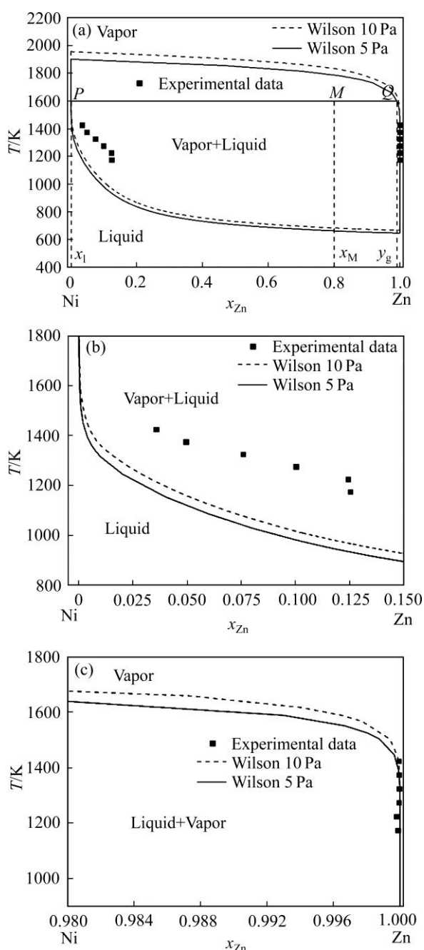
图3 5~10 Pa条件下Zn-Ni体系的 T - x - y 相图
