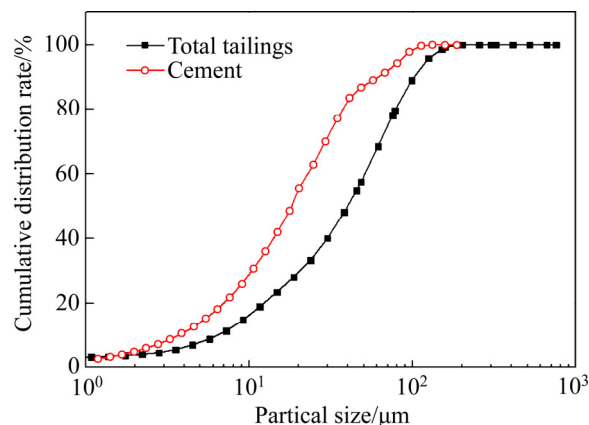
图 1 尾砂和水泥的粒径分布
