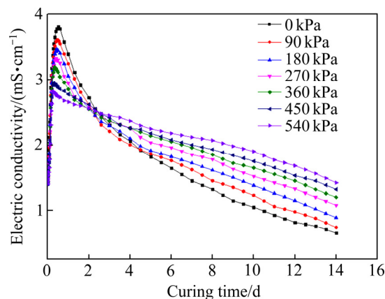
图 13 膏体充填体电导率与养护压力关系曲线
