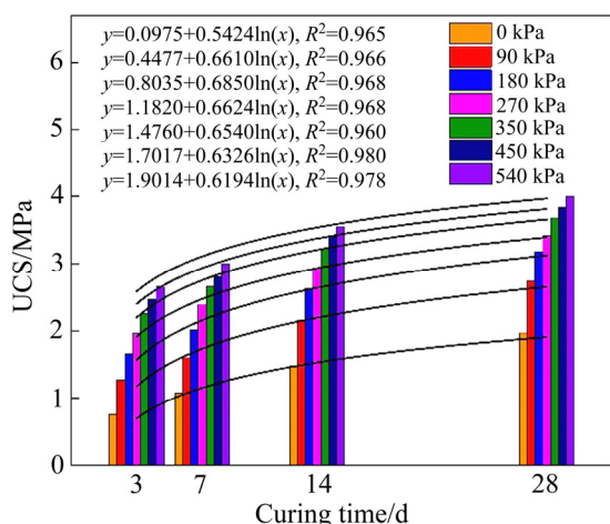
图 4 膏体充填体强度与养护时间的关系
