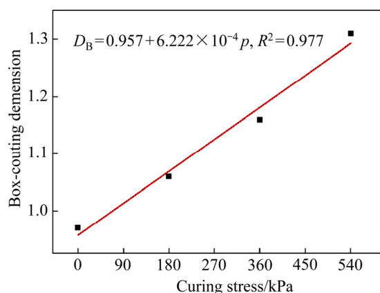
图 10 计盒维数与养护压力关系变化规律
