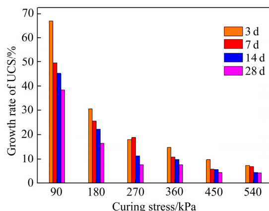
图 5 膏体充填体强度增长率随养护时间、养护压力变化规律
