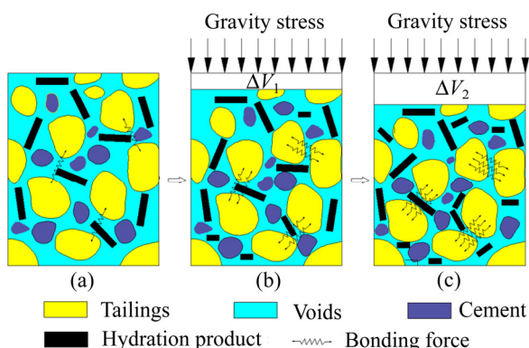
图 11 养护压力作用对膏体充填体强度影响机理分析图
