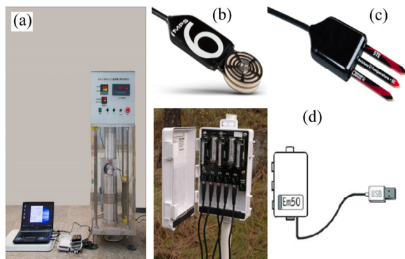
图2 膏体充填体多场耦合养护试验装置
