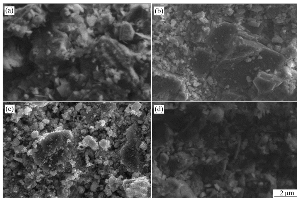
图 7 不同养护压力下膏体充填体的 SEM 像
