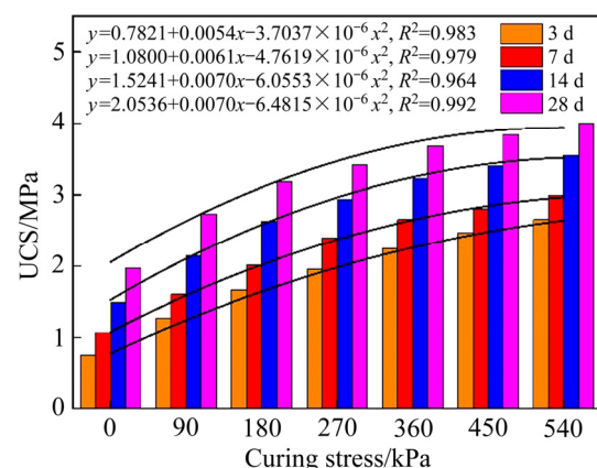
图 6 膏体充填体强度与养护压力的关系
