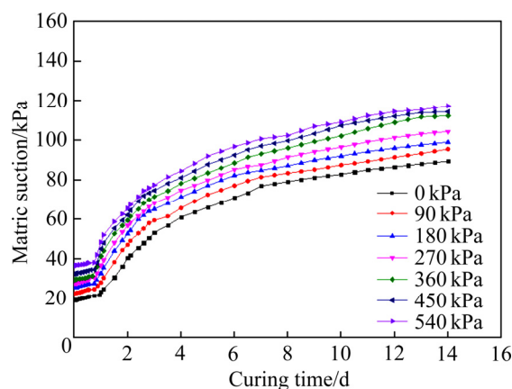
图 12 膏体充填体基质吸力与养护时间的关系
