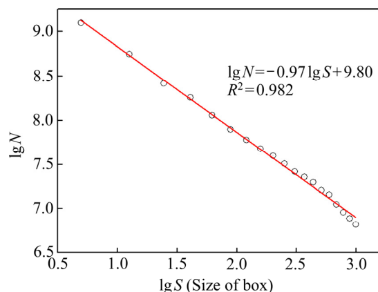
图 9 养护压力为 0 kPa 的膏体充填体分形维数
