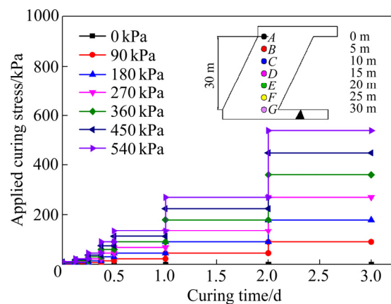
图3 膏体充填体养护过程中施加养护压力变化图
