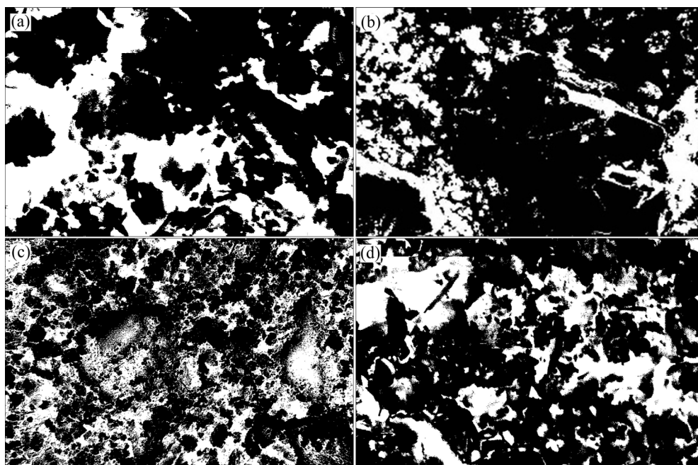
图 8 膏体充填体电镜扫描二值化图像
