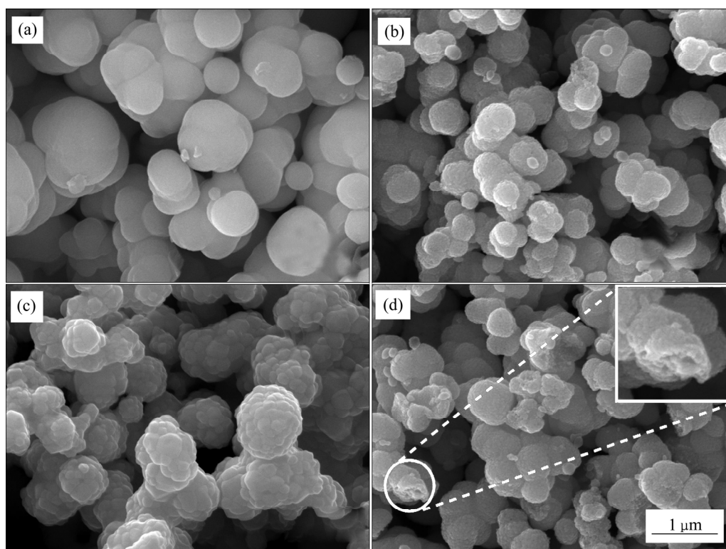
图3 前驱体和不同热处理时间所获 \text{Bi}_2\text{O}_3@\text{ZnO} 材料的 SEM 像
