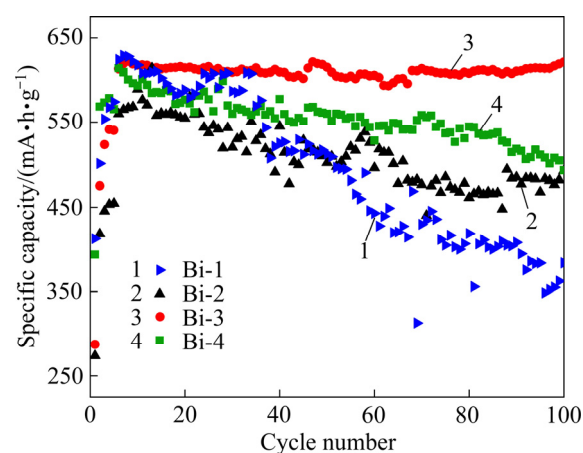
图 6 不同 Bi 含量 \text{Bi}_2\text{O}_3@\text{ZnO} 复合材料用于锌负极的循环性能
