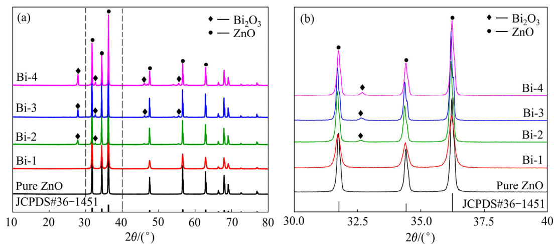
图4 不同 Bi 含量的 \text{Bi}_2\text{O}_3@\text{ZnO} 复合材料的 XRD 谱
