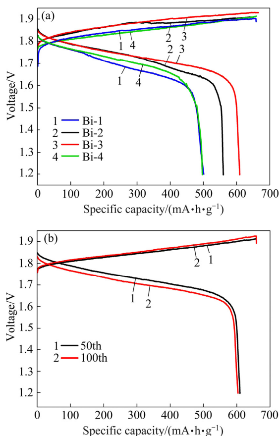
图 9 不同 Bi 含量 \text{Bi}_2\text{O}_3@\text{ZnO} 复合材料用于锌负极的第 50 圈充放电曲线以及 Bi-3 在第 50 圈和 100 圈的充放电曲线
