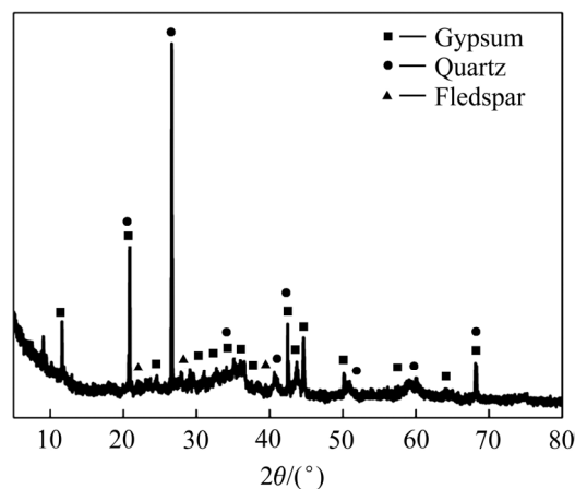
图 10 浸出渣 XRD 谱
