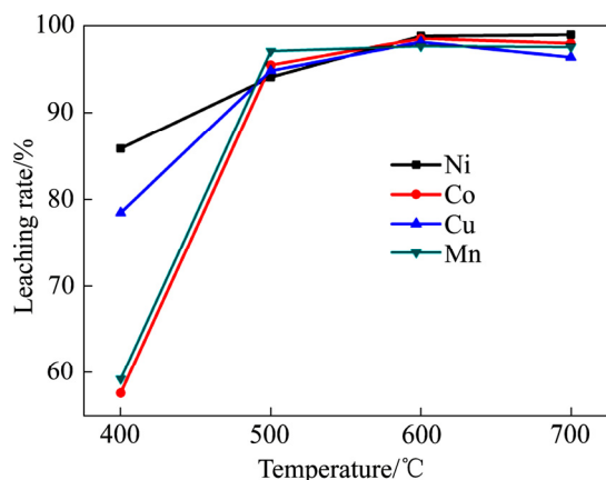
图 2 还原温度对有价值金属浸出率的影响
