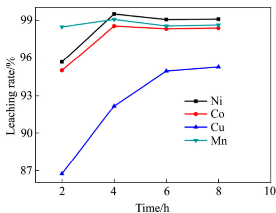
图 9 浸出时间对有价值金属浸出率的影响
