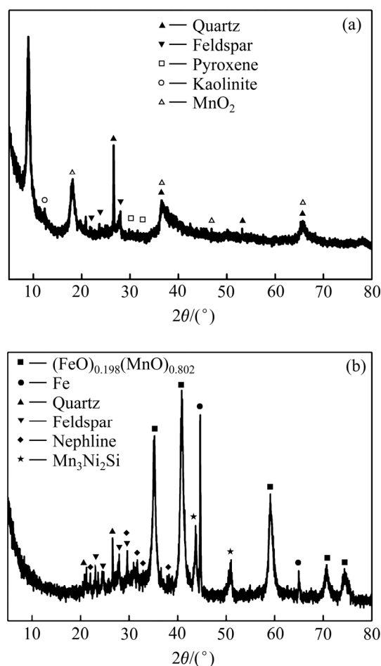
图 3 多金属结核及其 600 °C 氢还原物料 XRD 谱
