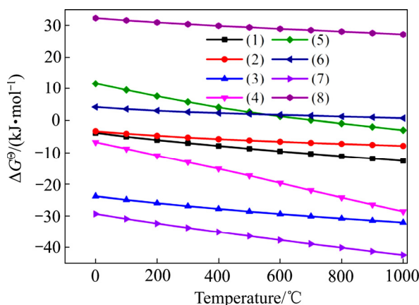
图 1 反应式(1)~(8)在不同温度下的吉布斯自由能
