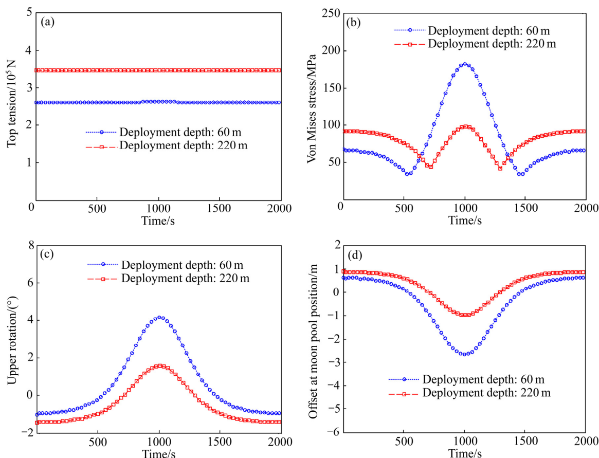
图8 内波上层流方向与海流反向工况的冲击响应
