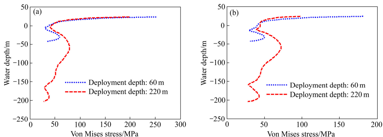
图 9 Von Mises 等效应力分布
