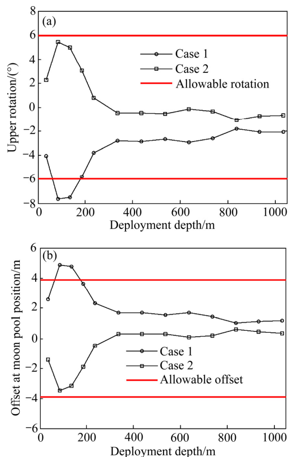
图13 上部转角和月池处偏移随布放深度的变化情况
