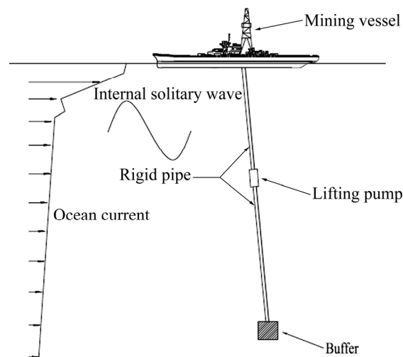
图1 中间仓收放系统组成示意图
