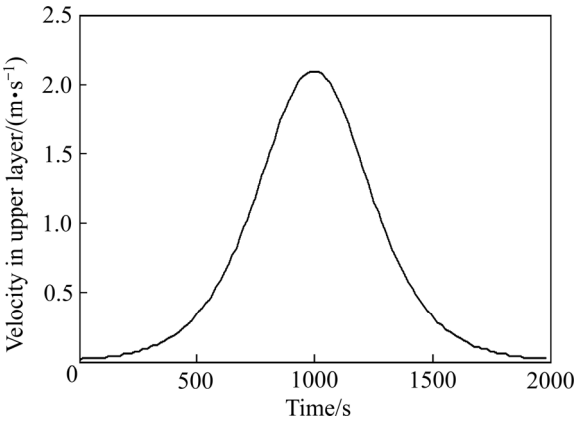
图 5 内波上层流速随时间的变化 Fig. 5 Change of internal wave velocity in upper layer with time
