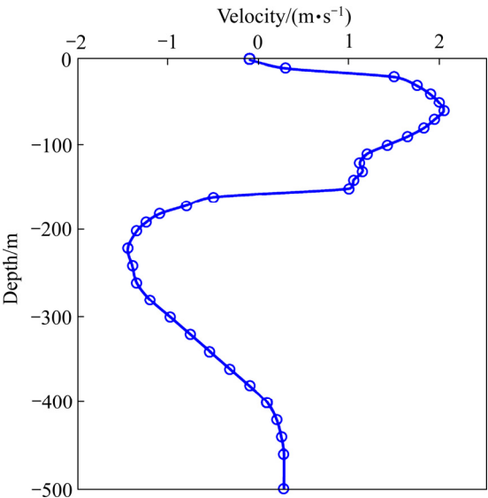
图 4 内波流速剖面 Fig. 4 Internal wave velocity profile
