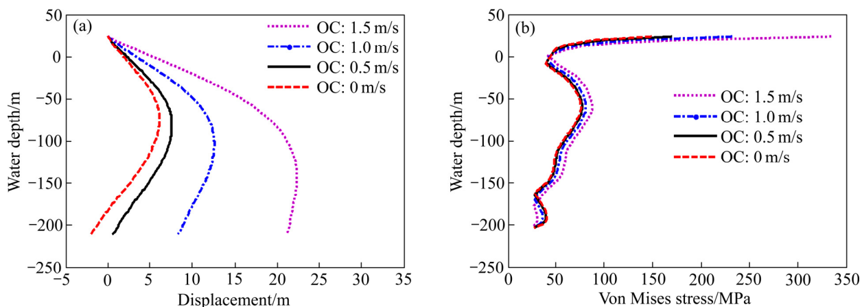
图 11 叠加不同强度海流的管柱形态与等效应力对比
