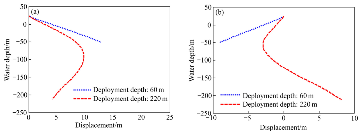
图 10 管柱形态变化
