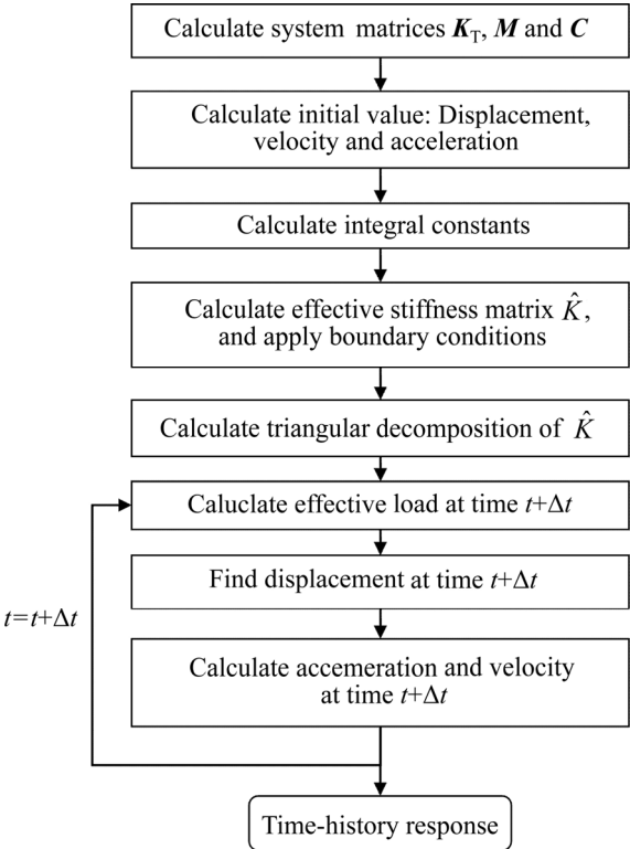
图 2 Newmark 积分算法流程 Fig. 2 Algorithm flow chart of Newmark- \beta method
