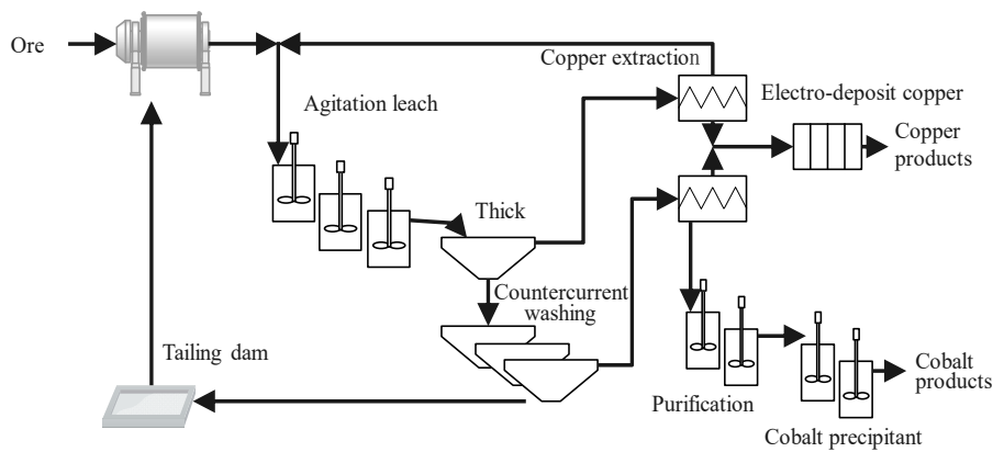
图 4 铜钴硫化矿分步浸出-萃取-电积流程
