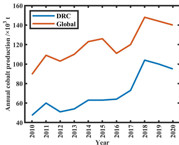
图3 刚果（金）钴资源历史年产量 [10]
