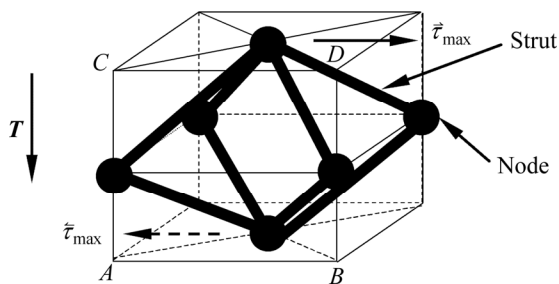
图3 扭矩作用下的多孔体圆轴内部孔隙单元受力分析模型
