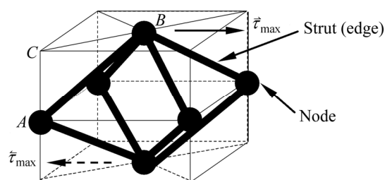
图 2 剪切载荷作用下多孔体中孔隙单元的受力分析模型
