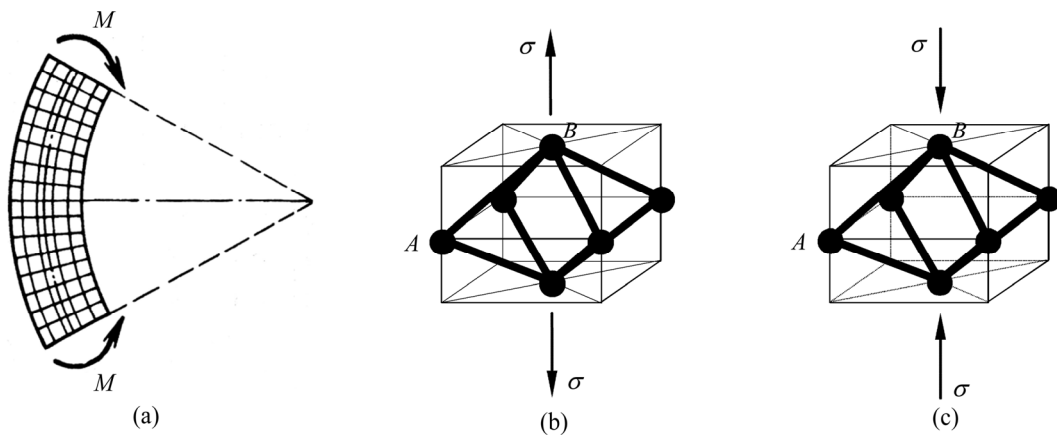
图4 弯矩作用下多孔体中孔隙单元的受力分析模型
