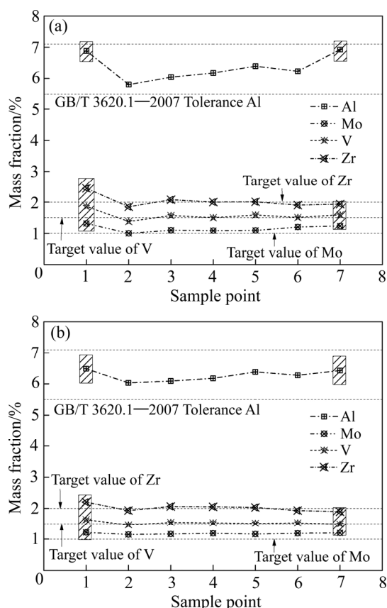
图 5 TA15 合金铸锭轴向化学成分分布
