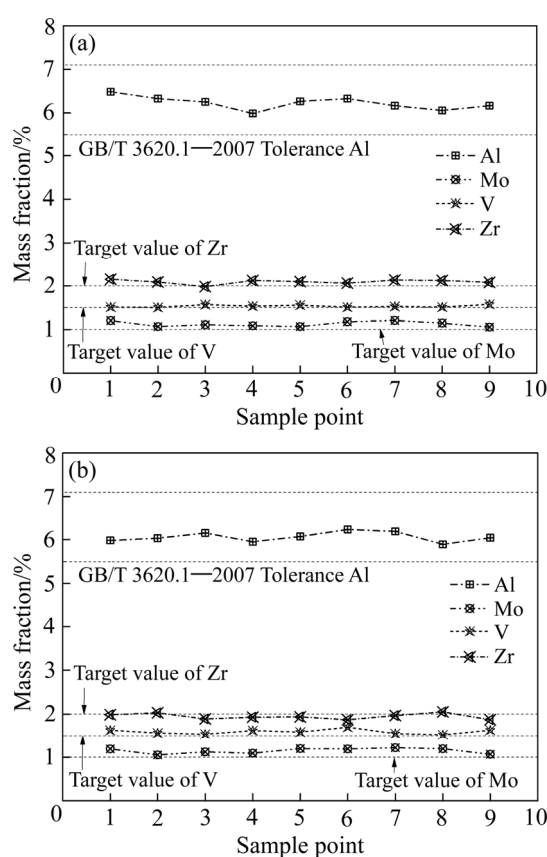
图 6 1 号铸锭横截面化学成分分布
