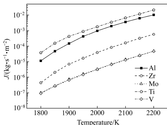
图 4 TA15 钛合金各元素的自由挥发速率与温度的关系
