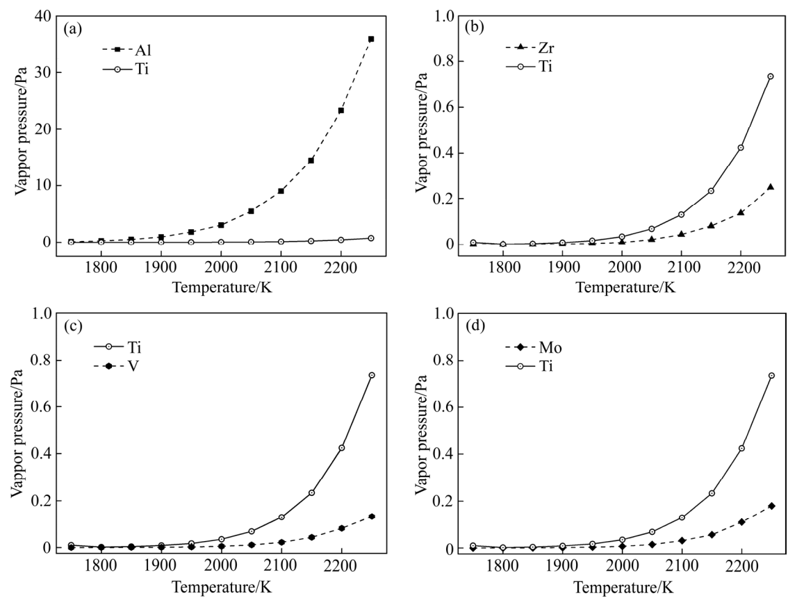
图 3 TA15 钛合金熔体中各元素的饱和蒸气压和温度的关系
