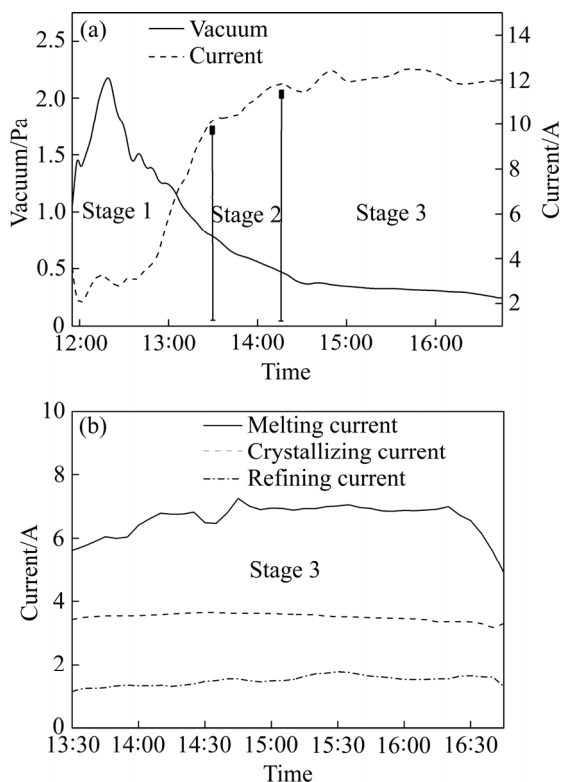
图2 熔炼工艺参数变化曲线
