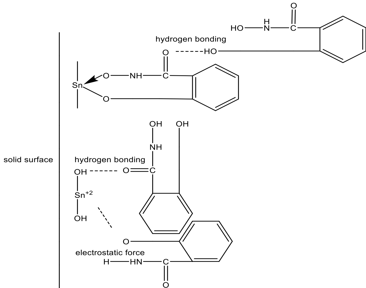
图5 水杨羟肟酸 (SHA) 与锡石作用吸附机理图 [44]
