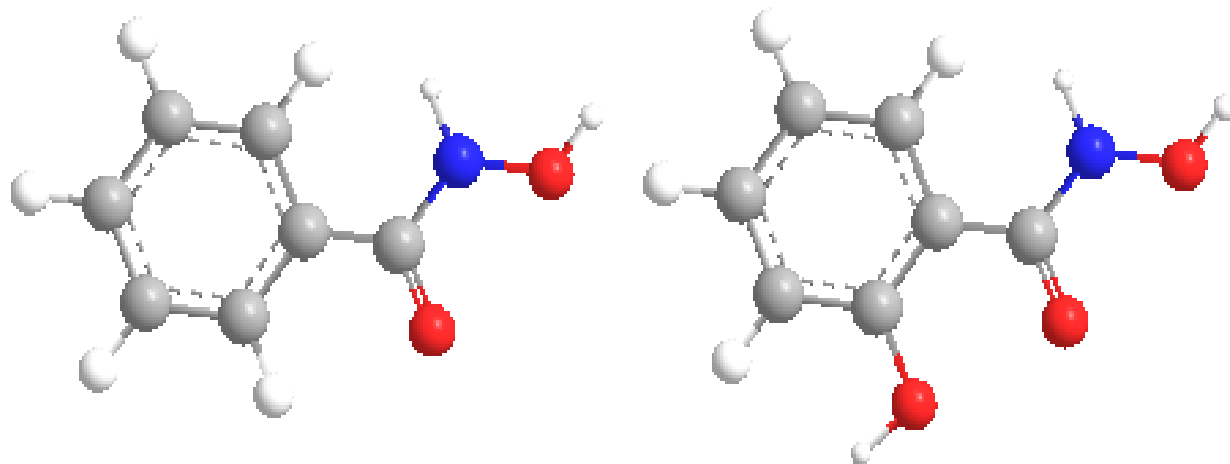
图 3 苯甲羟肟酸(左)、水杨羟肟酸(右)分子结构图
