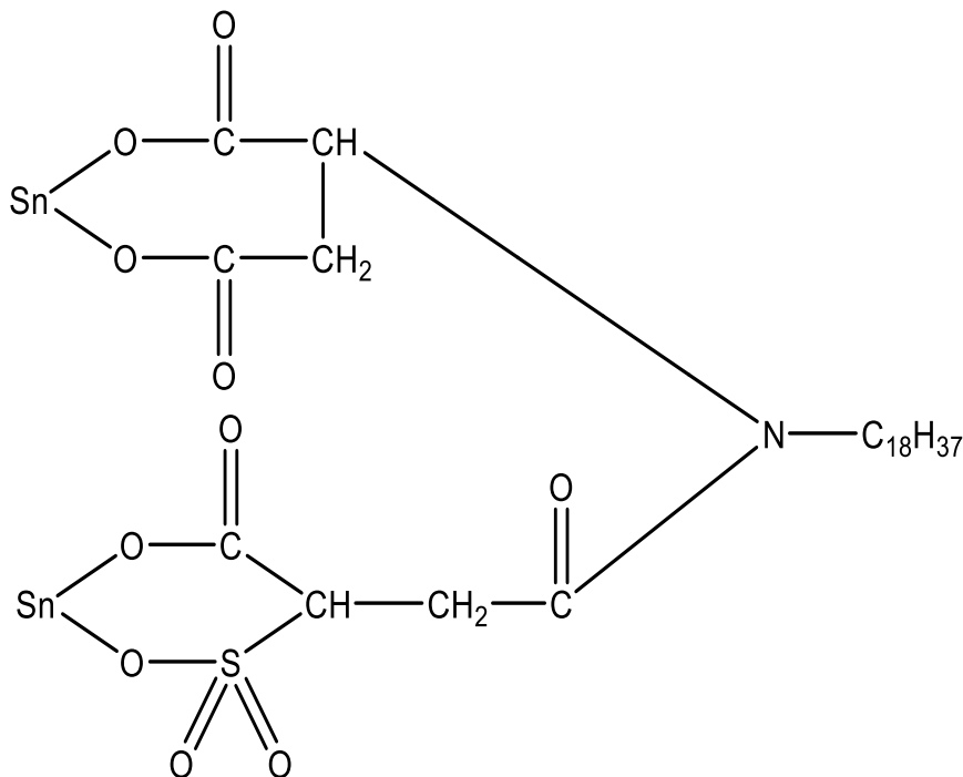
图 2 Aerosol-22 与锡石表面作用机理图 [34]
