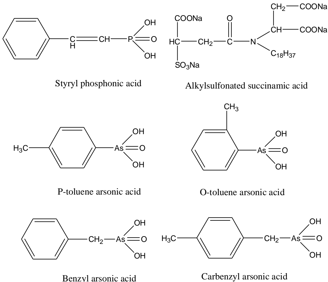
图 1 分子结构图
