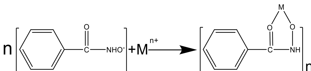
图 4 螯合反应结构示意图 [36]
